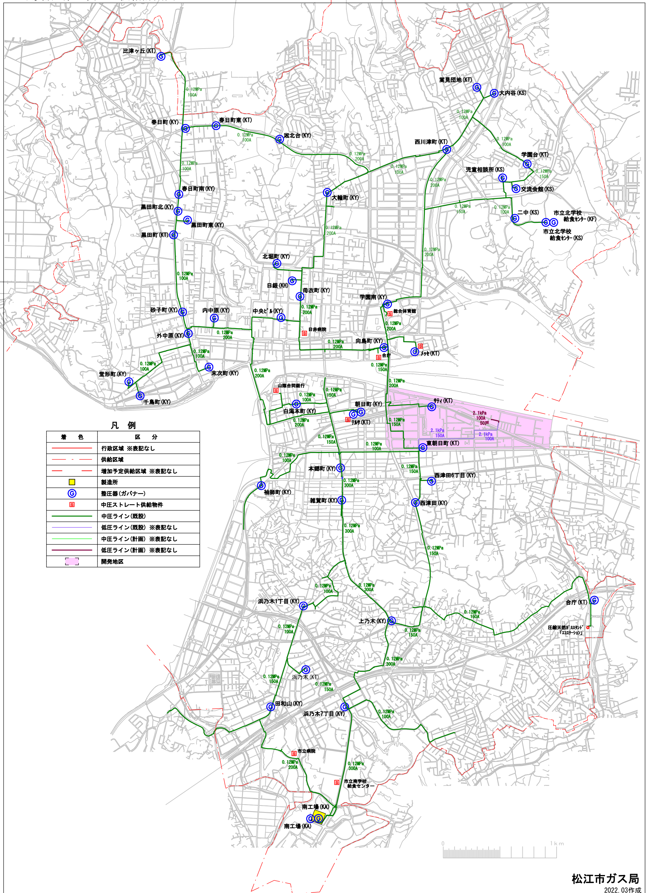
(導管) 第7表 供給計画図
